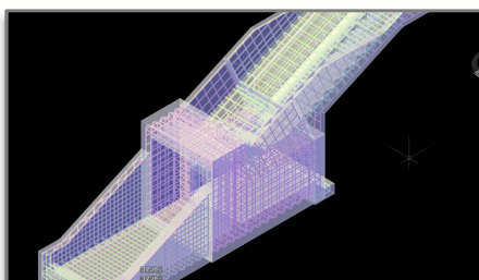
配筋の3次元化
